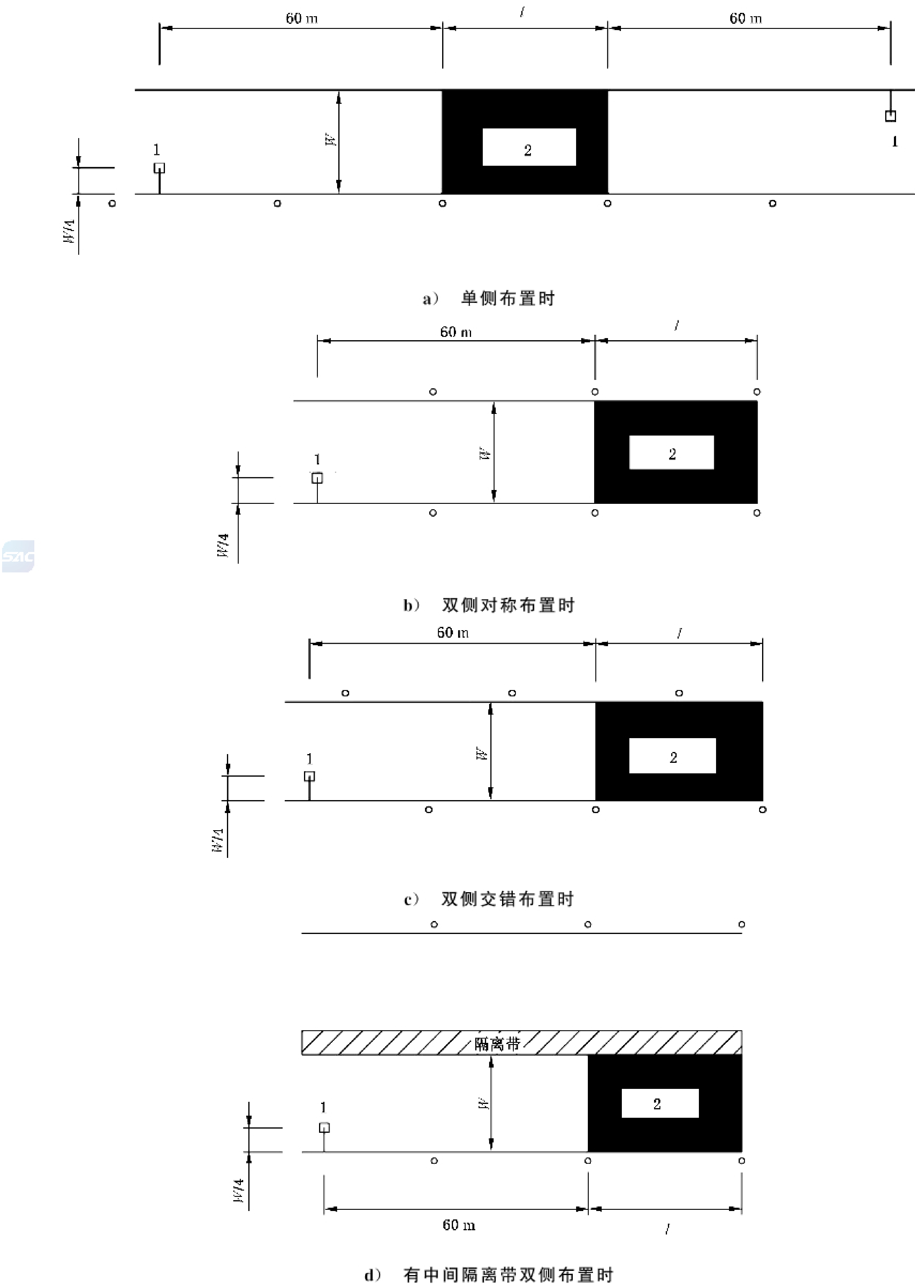
图 8 道路亮度测量时亮度计的观测点示意图
