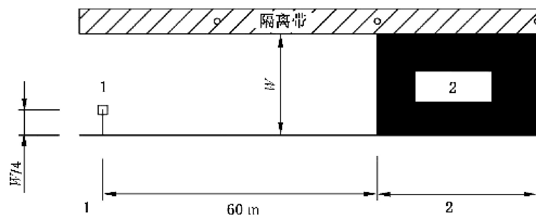
e) 有中间隔离带中心对称布置时
