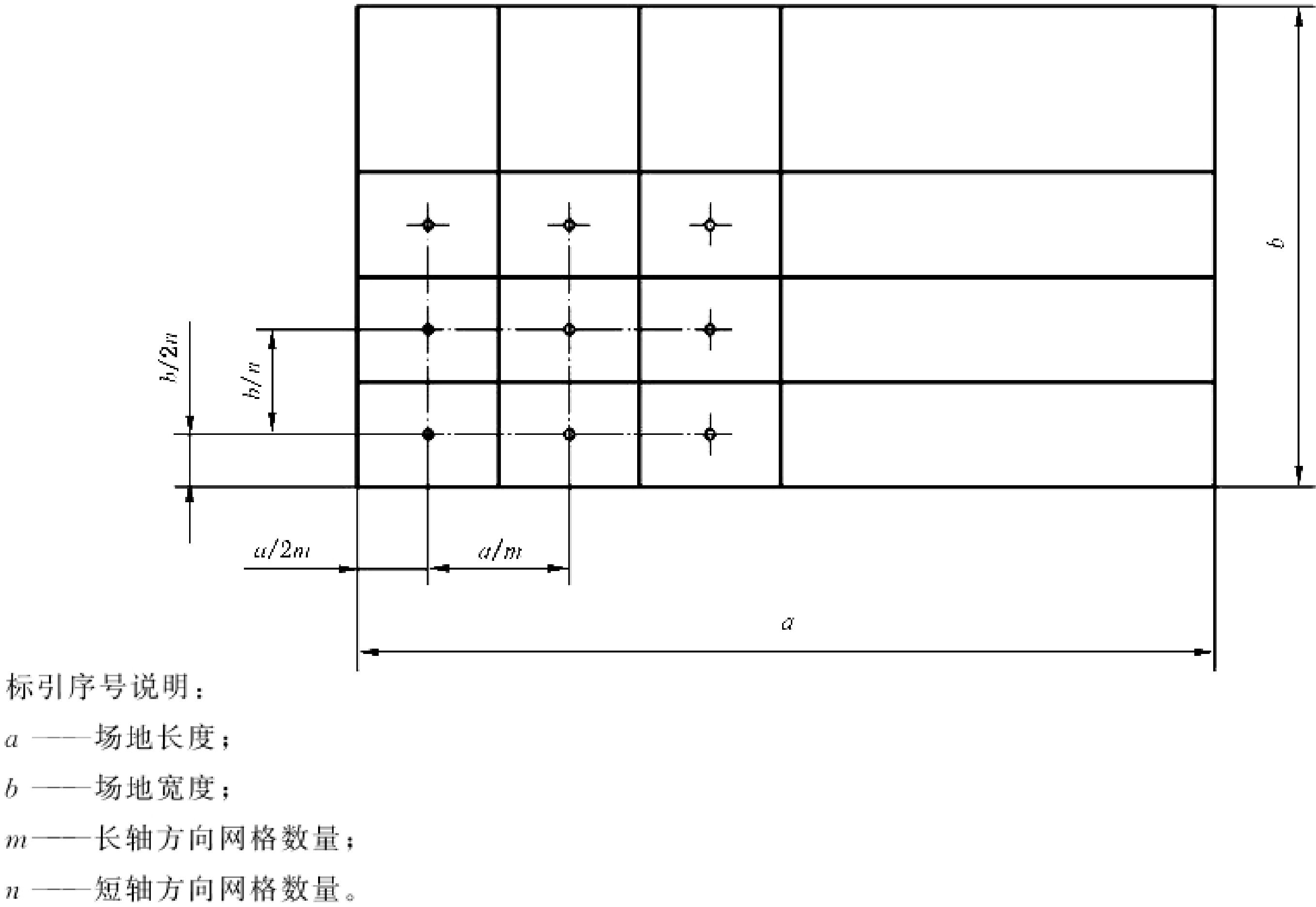
图 1 在网格中心布点示意图
