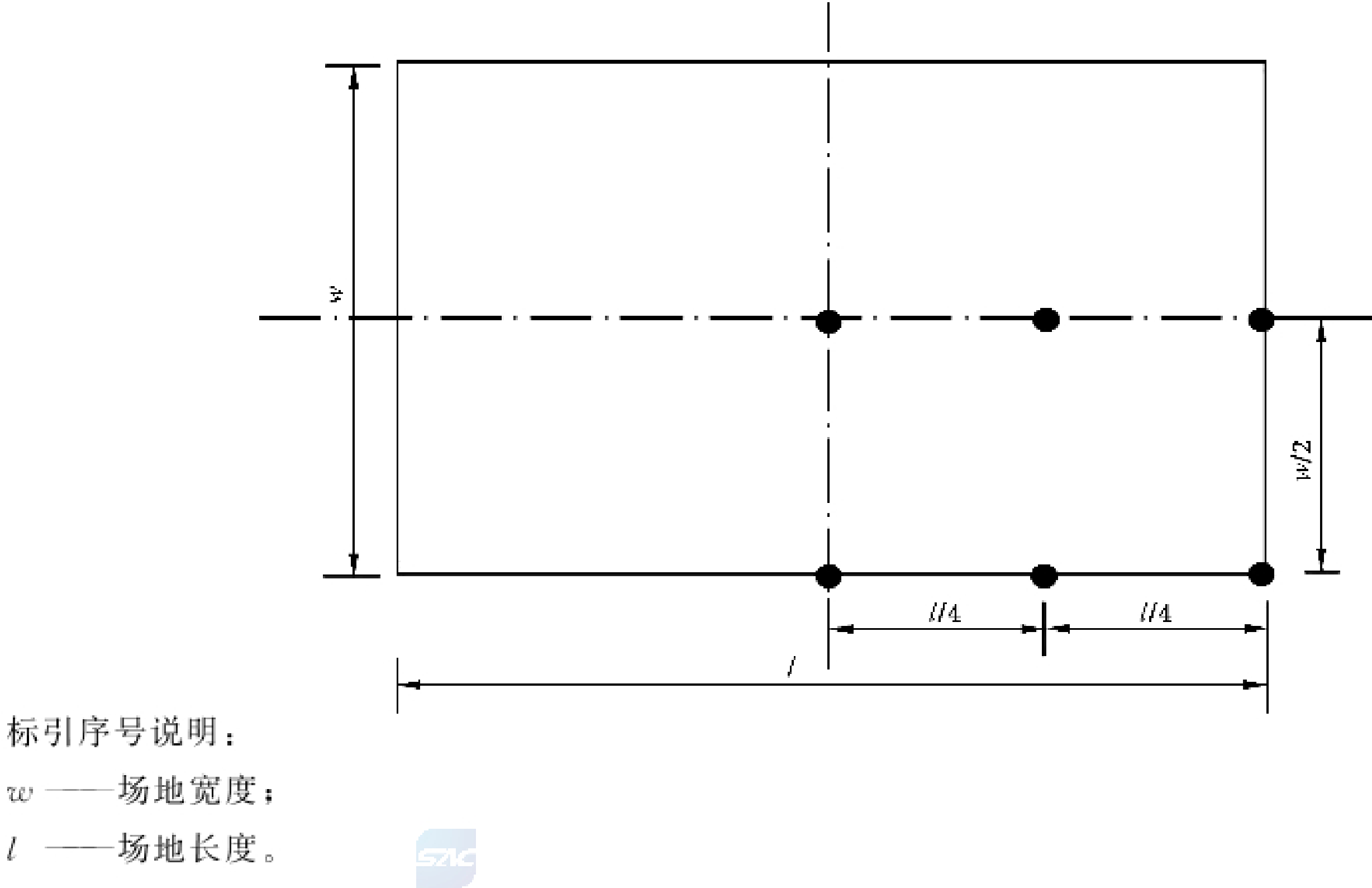
图 9 公园、广场眩光值测点图
